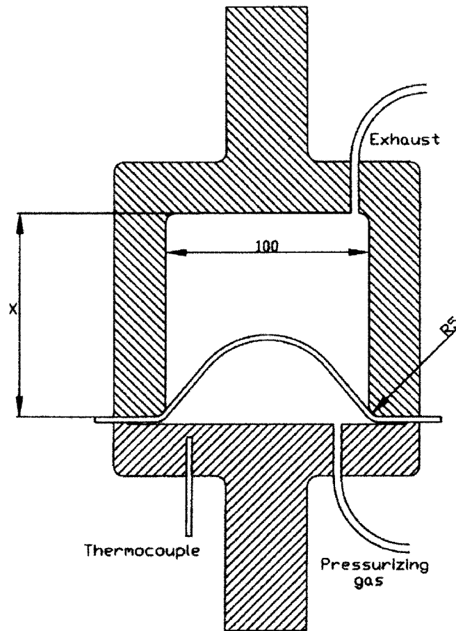
FIG. 1 Bulge-Forming Apparatus
