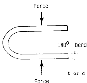
FIG. 12 Type 1 180° Free Bend
