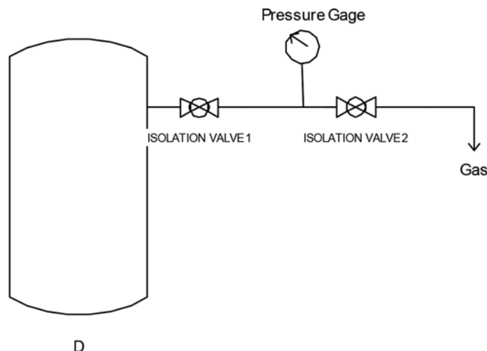
FIG. 1 Test Apparatus
