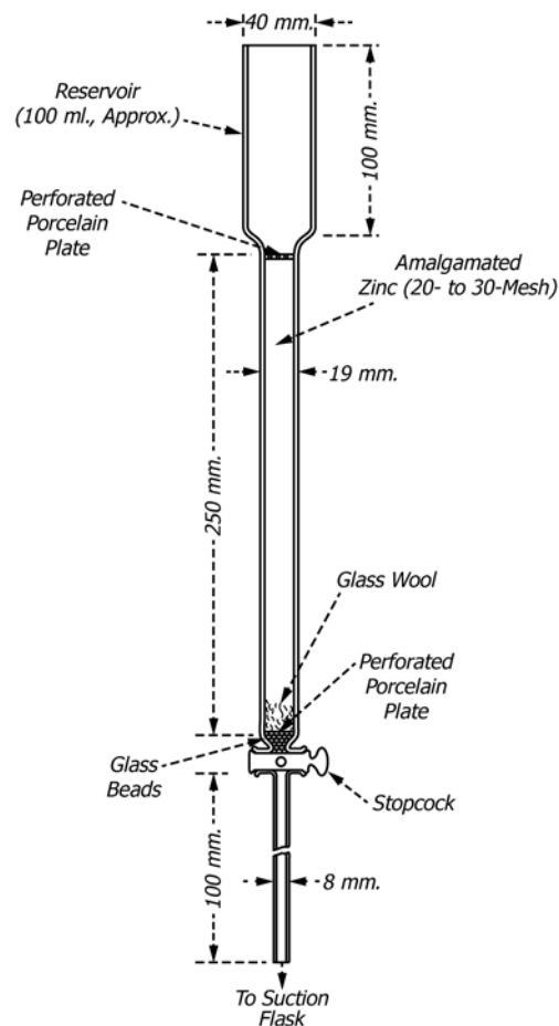
FIG. 4 Jones Reductor
