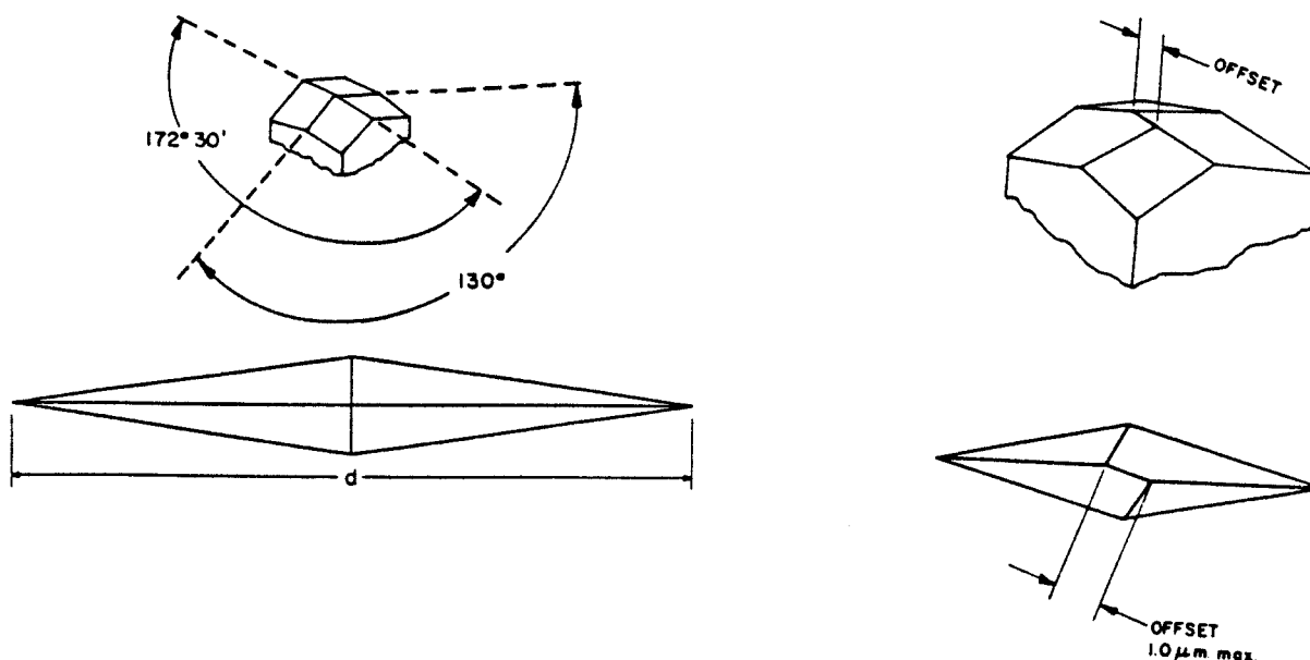
FIG. 1 Knoop Indenter
