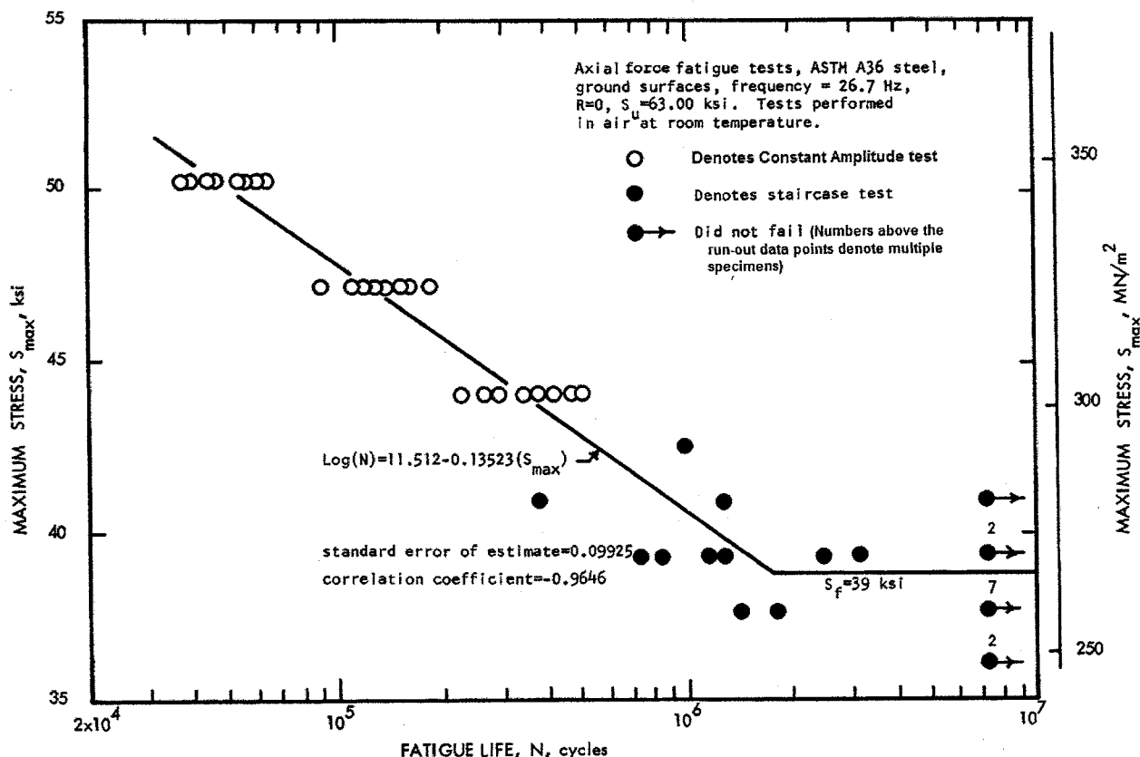
FIG. 1 S-N Diagram
