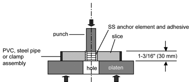
FIG. 12 Punch Test
