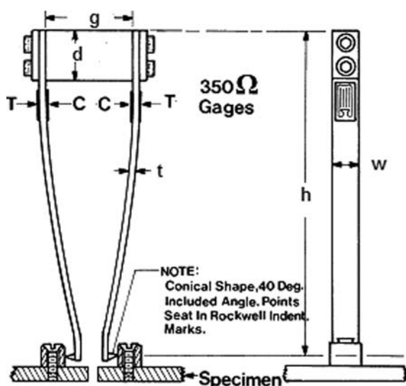
Dimensions
