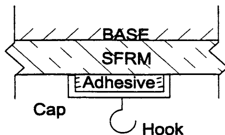
FIG. 2 In-Place Apparatus
