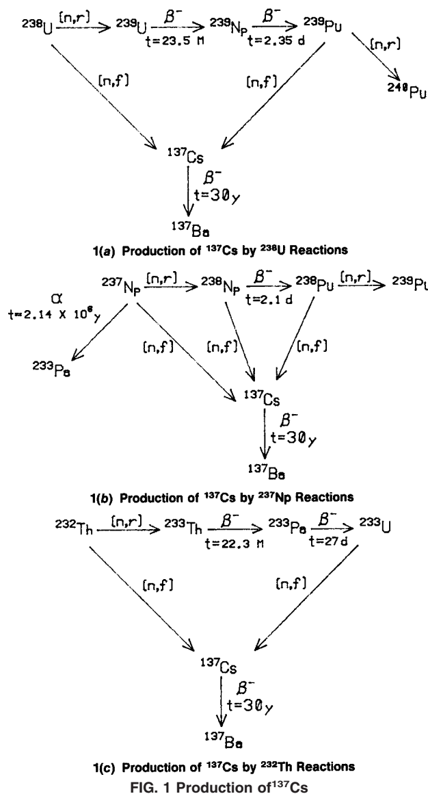
FIG. 1 Production of ^{137}\text{Cs}
