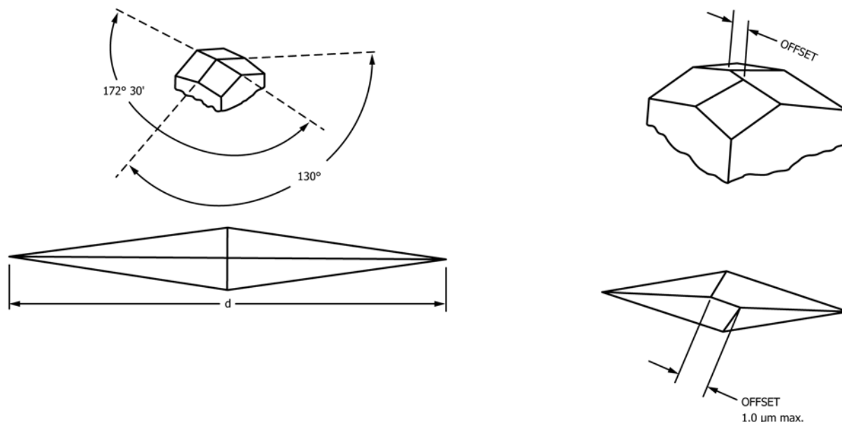
FIG. 2 Knoop Indenter
