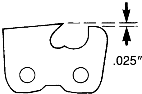
FIG. A1.13 Depth Gage
