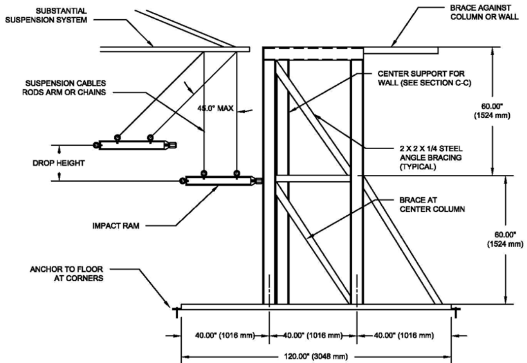
FIG. 4 Test Wall
