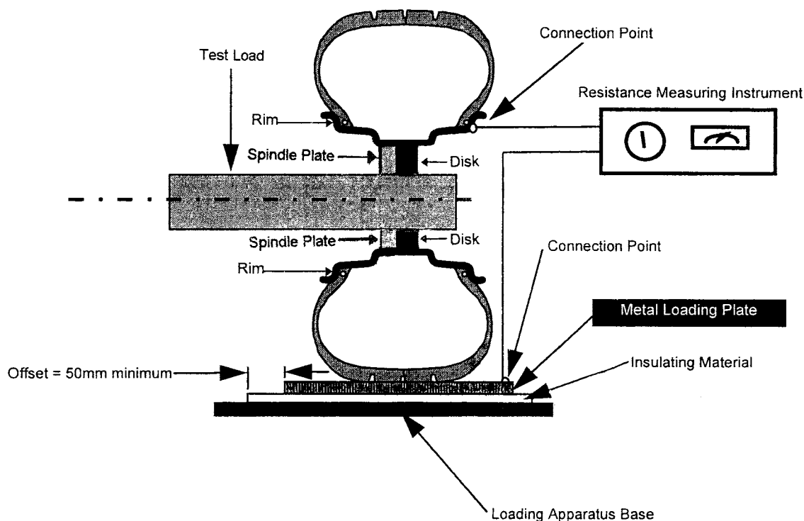
FIG. 1 Apparatus
