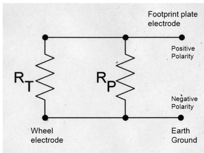
FIG. 1 Apparatus
