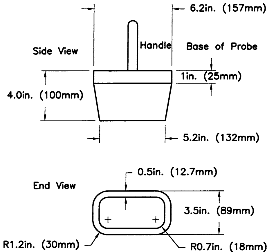
FIG. 2 Torso Probe
