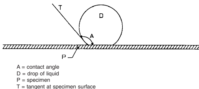
FIG. 1 Contact Angle
