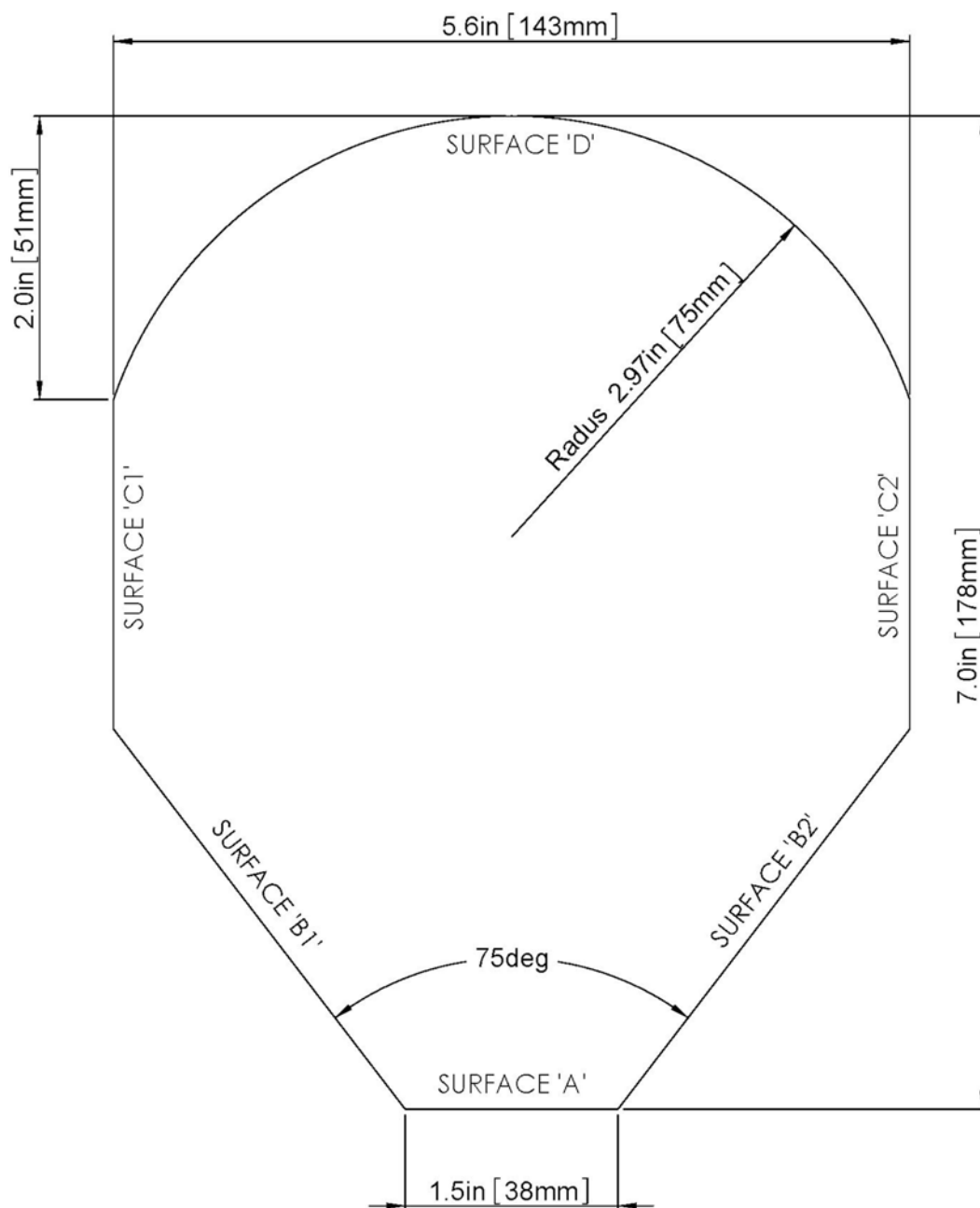
FIG. A1.36 Test Template B
