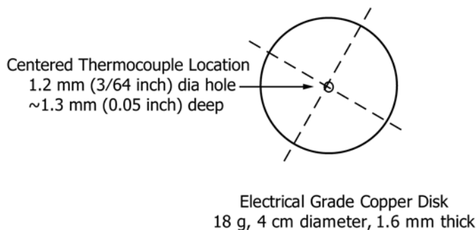
FIG. 5 Calorimeter
