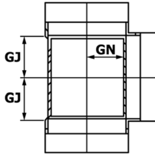
FIG. X1.4 Vent Tee
