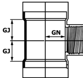
FIG. X1.7 Cleanout Tee
