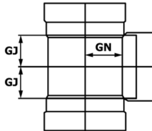
FIG. X1.4 Vent Tee
