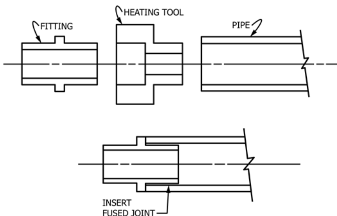
FIG. 7 Insert Fusion
