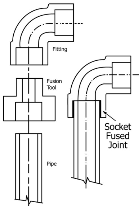
FIG. 6 Socket Fusion
