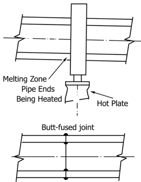
FIG. 3 Butt Fusion
