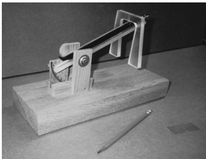
FIG. 1 Apparatus
