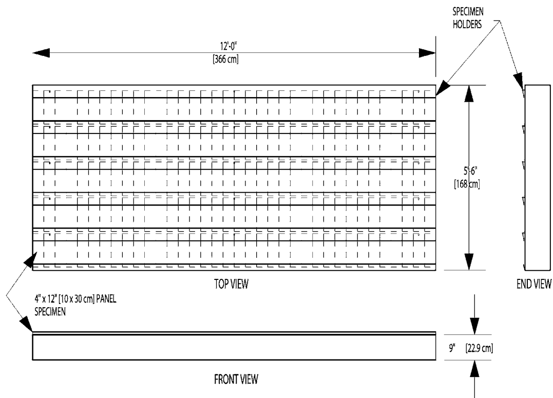
FIG. 3 Black Box
