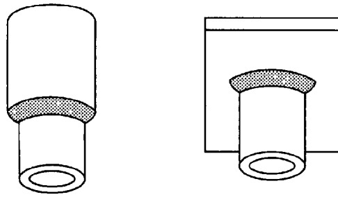
(D) OVERHEAD WELDING TEST POSITION—4F
