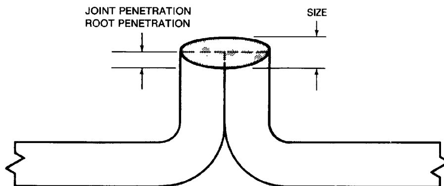
(H) EDGE WELD SIZE
