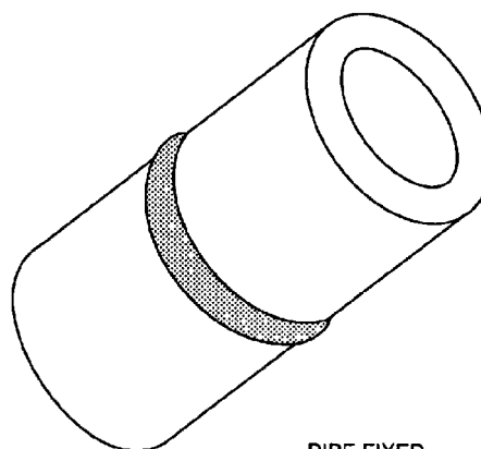
(D) MULTIPLE WELDING TEST POSITION—6GR
