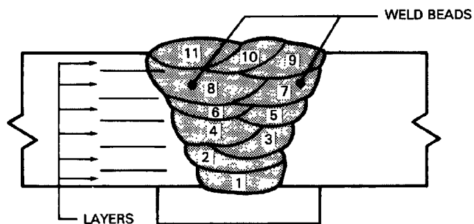
(D) CROSS-SECTIONAL SEQUENCE
