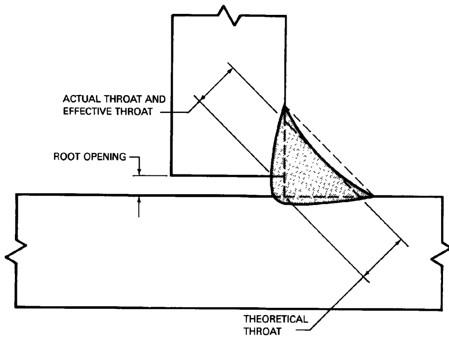
(D) T-JOINT WITH ROOT OPENING
