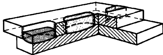
(D) SLOT WELDS
