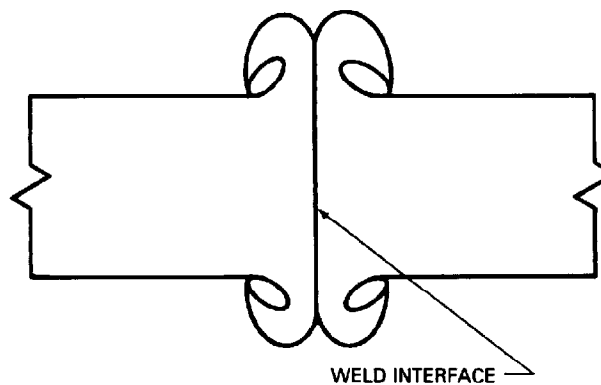
(D) FRICTION WELD
