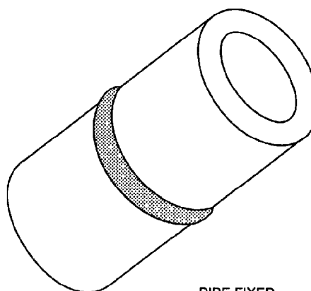
(D) MULTIPLE WELDING TEST POSITION—6G
