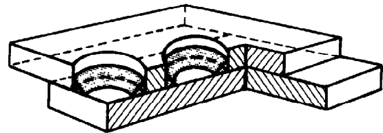
(F) FILLET WELDS
