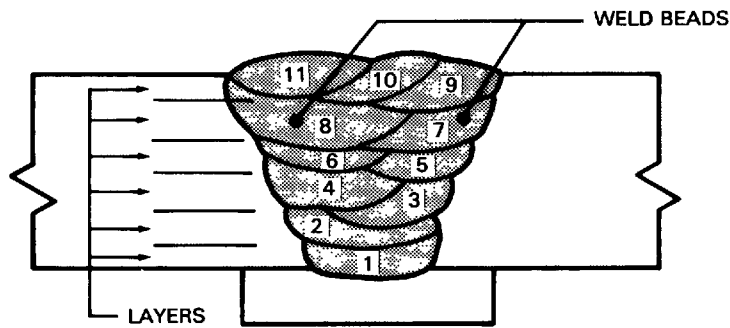
(D) CROSS-SECTIONAL SEQUENCE
