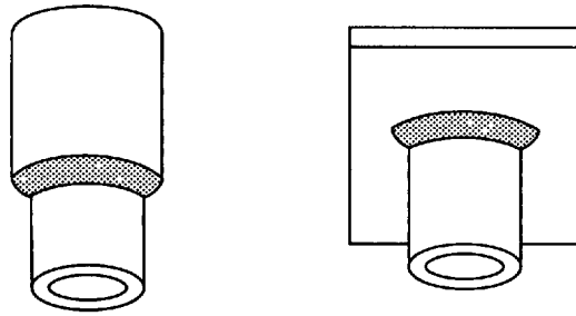
(D) OVERHEAD WELDING TEST POSITION—4F
