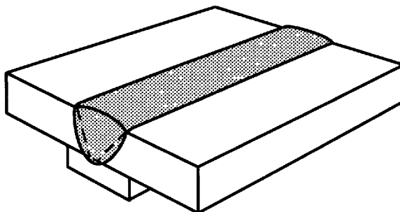
(D) SINGLE-V-GROOVE WELD WITH BACKING
