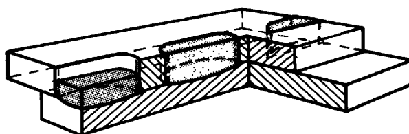
(D) SLOT WELDS
