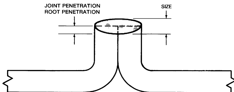
(H) EDGE WELD SIZE
