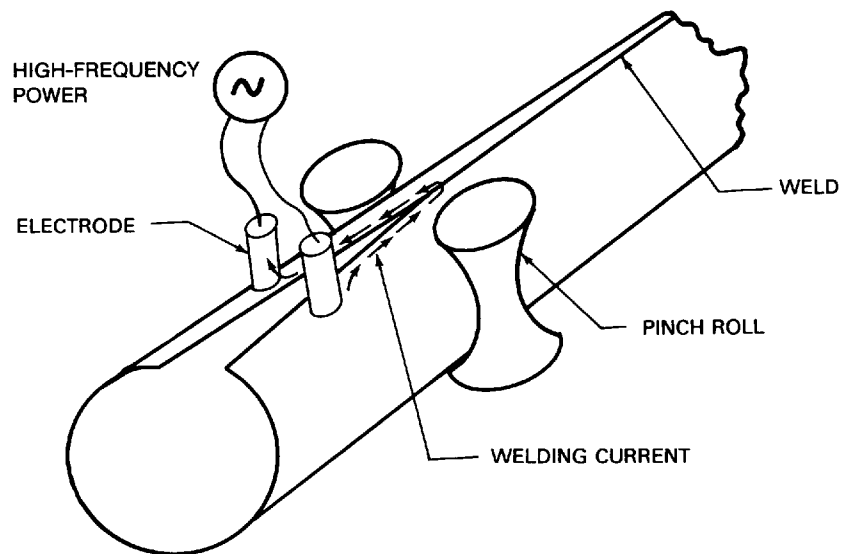
(D) HIGH FREQUENCY UPSET WELDING OF TUBE
