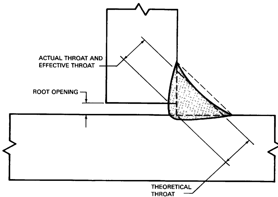
(D) T-JOINT WITH ROOT OPENING
