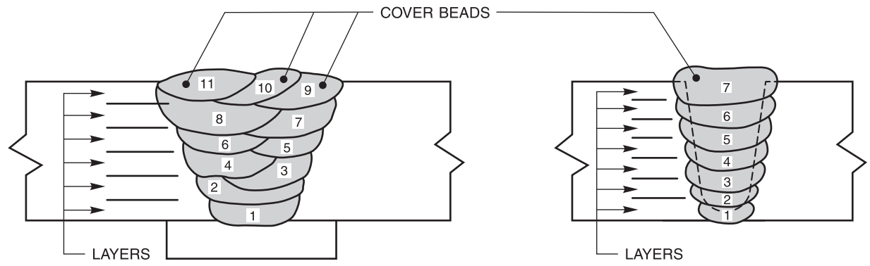
(D) CROSS-SECTIONAL SEQUENCE*
