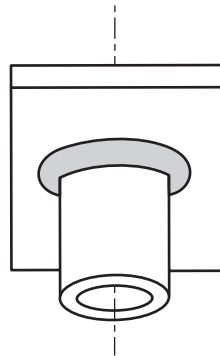
(D) OVERHEAD WELDING TEST POSITION—4F
