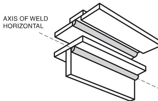
(D) TEST POSITION 4F (OVERHEAD)
