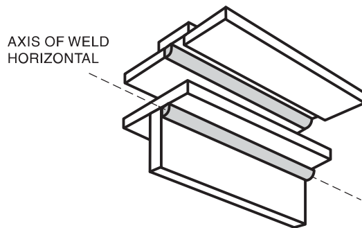
(D) TEST POSITION 4F (OVERHEAD)
