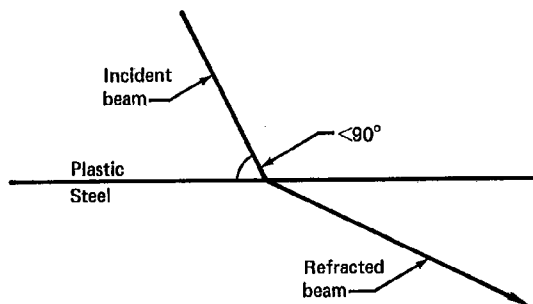
Fig. 19—Refraction
