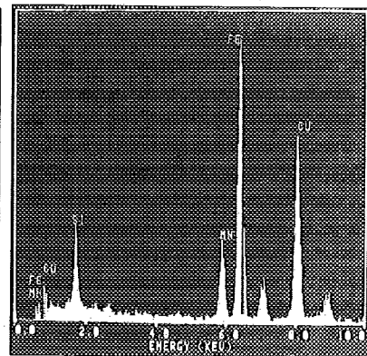
EDXA Spectrum
