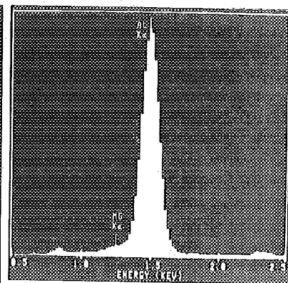
EDXA Spectrum
