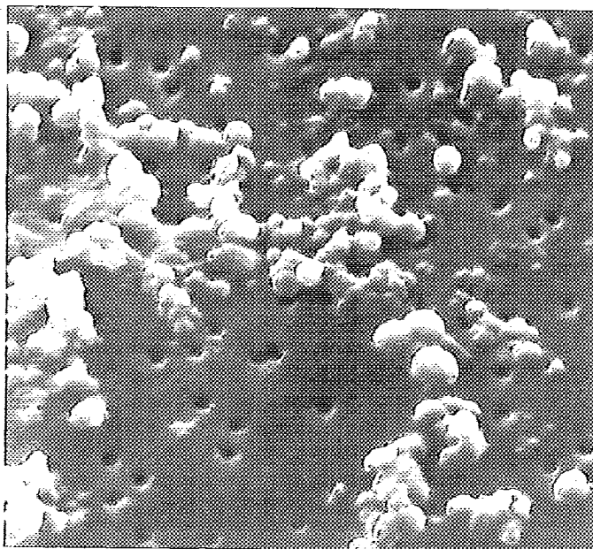
Fig. 1e — E70T-1 fume (20,000X)
