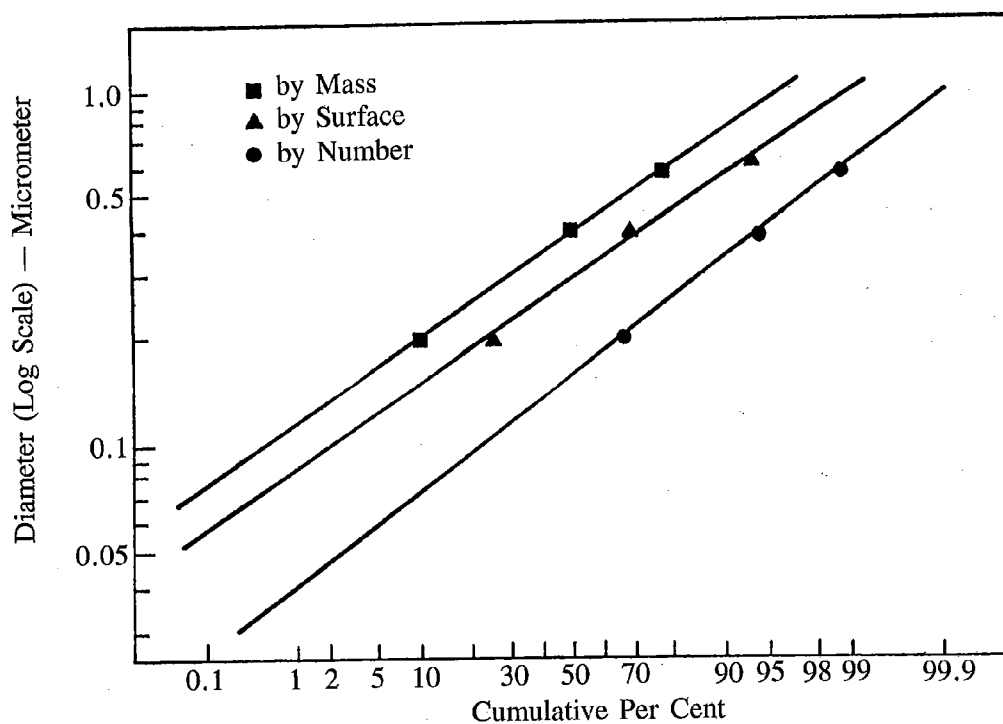
Fig. 5 — E7018
