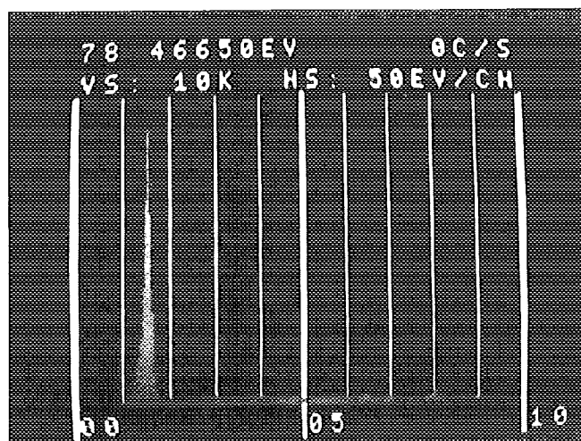
Fig. 2a — E6010 fume
