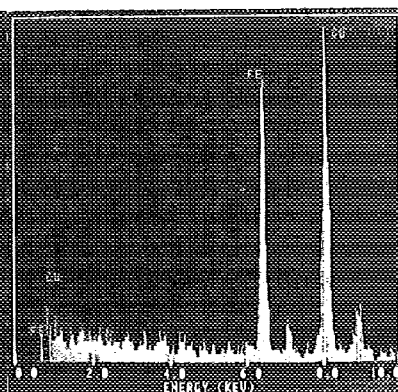
EDXA Spectrum
