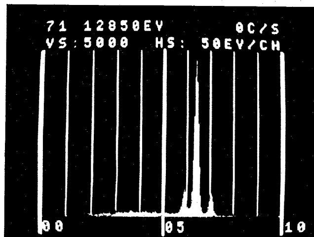
Fig. 2c — E7018 fume
