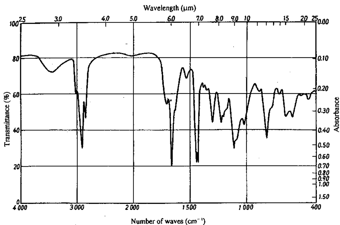
Annex 2 Fig. 1-4 Chloroprene rubber
