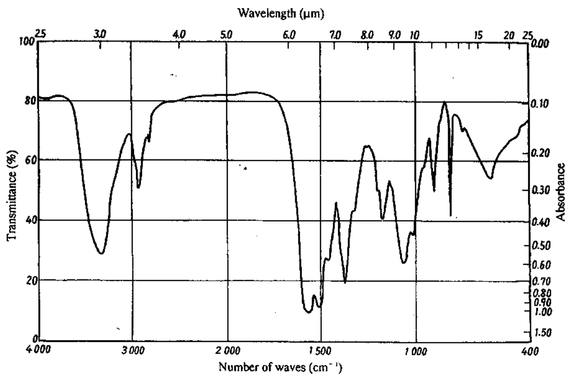
Annex 2 Fig. 9 Melamine
