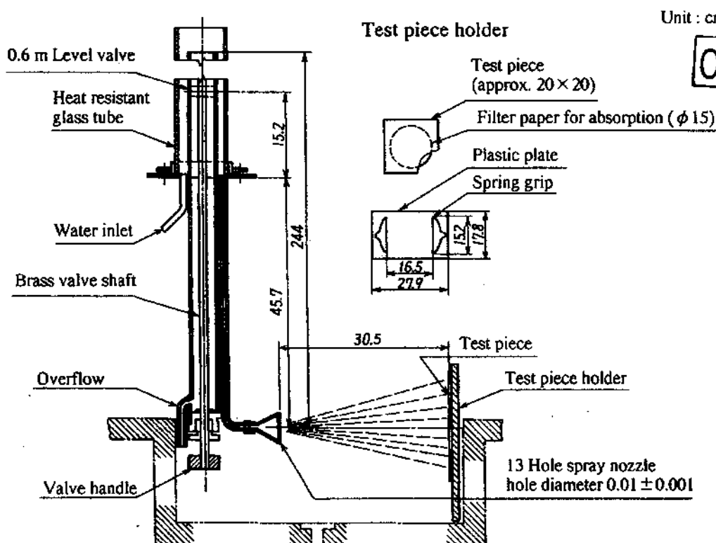
Annex 3 Fig. 1 Rain tester
