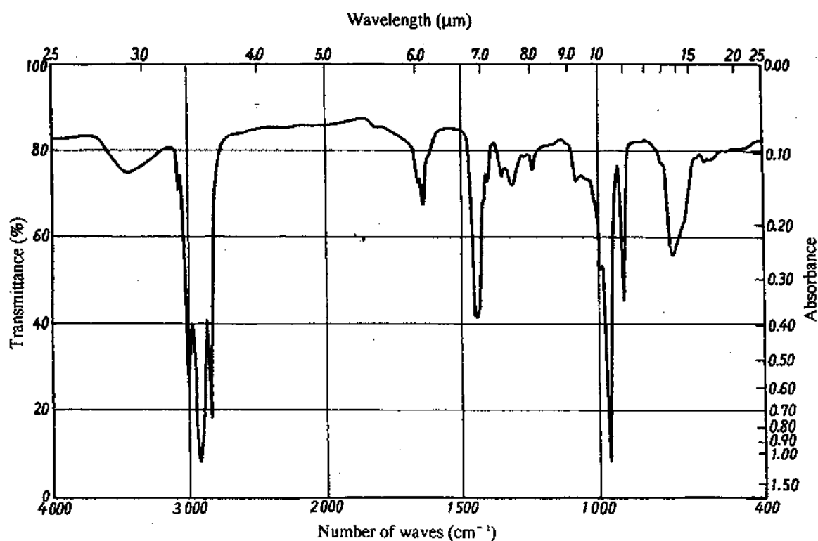
Annex 2 Fig. 1-2 Butadiene rubber
