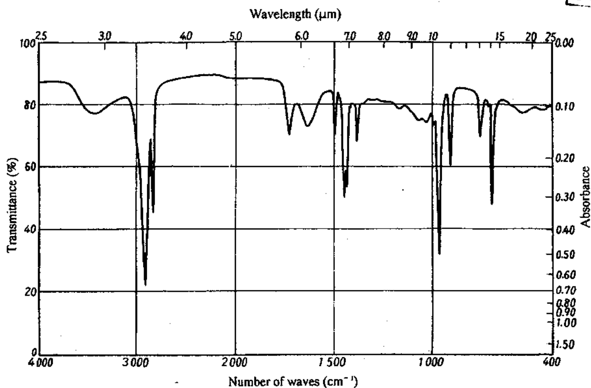
Annex 2 Fig. 1-3 Styrene-butadiene rubber
