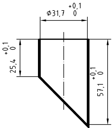
Figure 7 — Cylindre d'essai pour petits éléments
