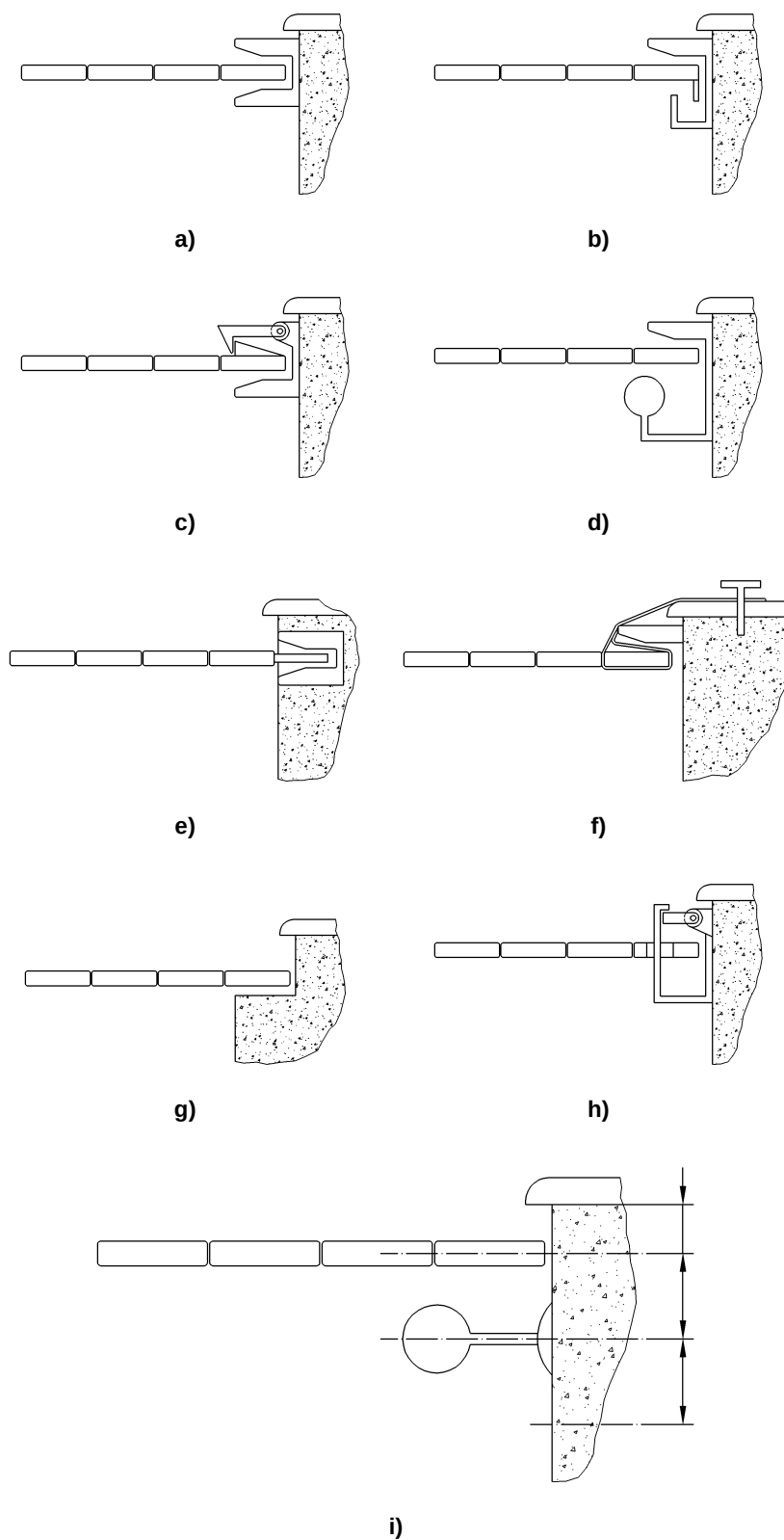
Figure 14 — Exemples de dispositifs de maintien des lames
