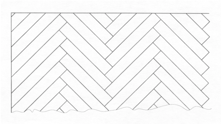
Figure 14 — "Herringbone" parquet flooring / Parquet "à bâtons rompus" / Fischgrätartig verlegter Parkettboden
