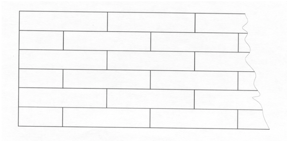
Figure 13 — Brick-pattern parquet flooring / Parquet "à coupe de pierre" / Parkettboden riemenartig im regelmäßigen Verband verlegt
