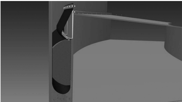
15. Foam seal (3).
