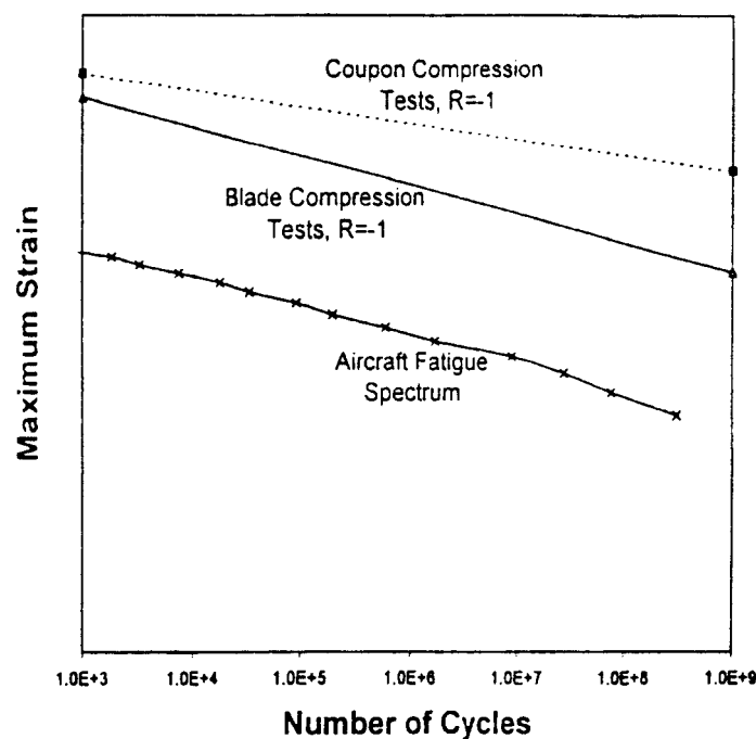
Figure 6.9. Fatigue data.
