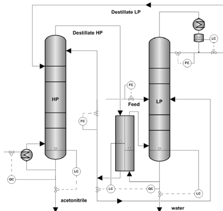
Fig. 5.17 Cascade controller.
