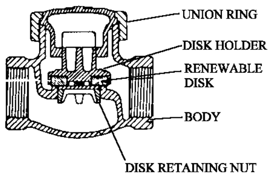
LIFT (DISK)
