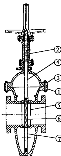
CONDUIT GATE
