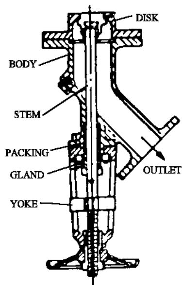
FLUSH BOTTOM
