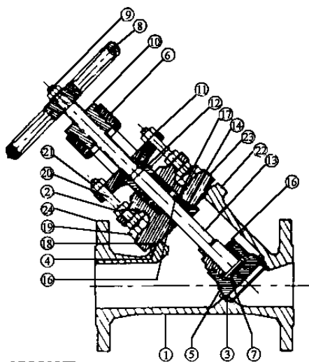
OBLIQUE
