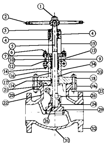
GLOBE ( BOLT TYPE DISK )
