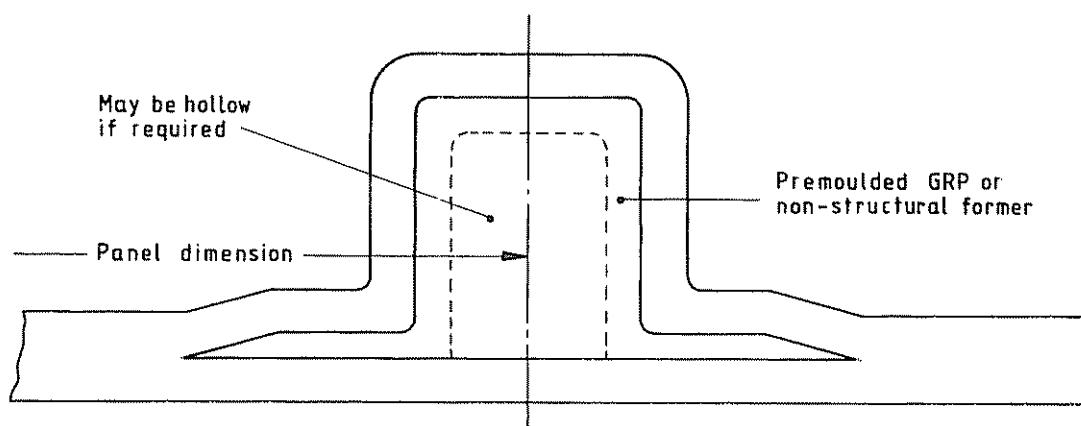
(d) GRP stiffener
