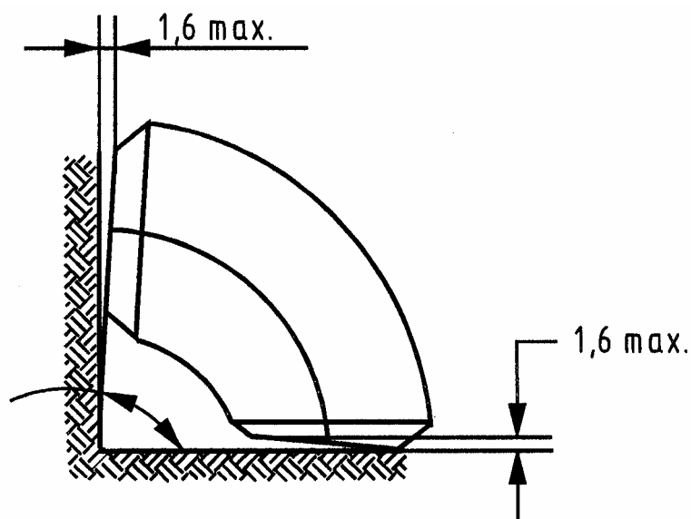
b) Bends
