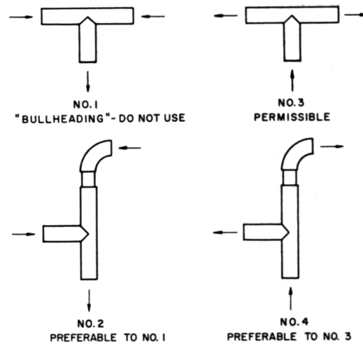
FIG. 5 — TEES
