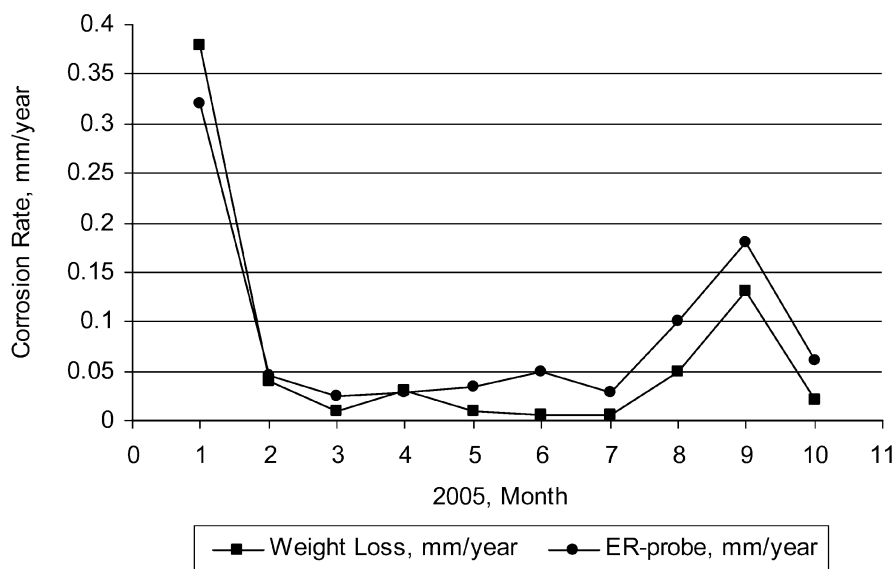
Fig. 5.11 Comparison ER and WL data.
