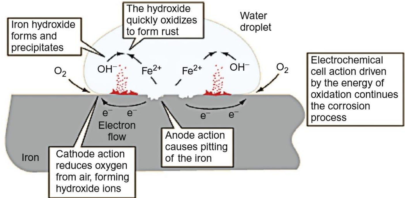
CUI of carbon steel
