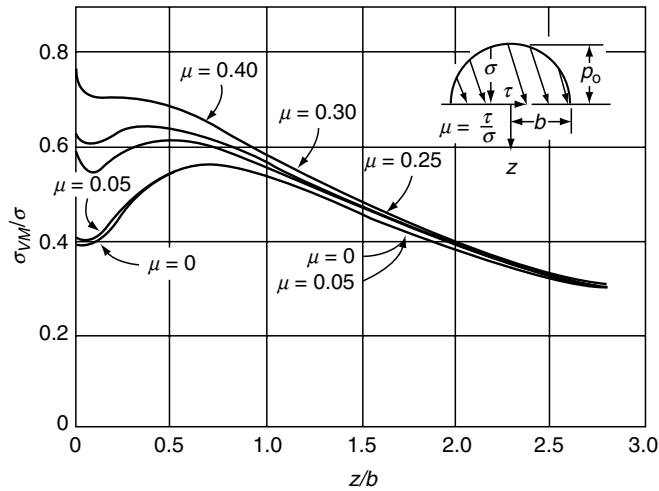
FIGURE 6.19 Material stressing ( \sigma_{VM}/\sigma ) vs. depth for different amounts of surface shear stress ( \tau/\sigma ). (From Zwirlein, O. and Schlicht, H., Werkstoffanstregung bei Wälzbeanspruchung-Einfluss von Reibung und Eigenspannungen , Z. Werkstofftech. , 11, 1–14, 1980.)
