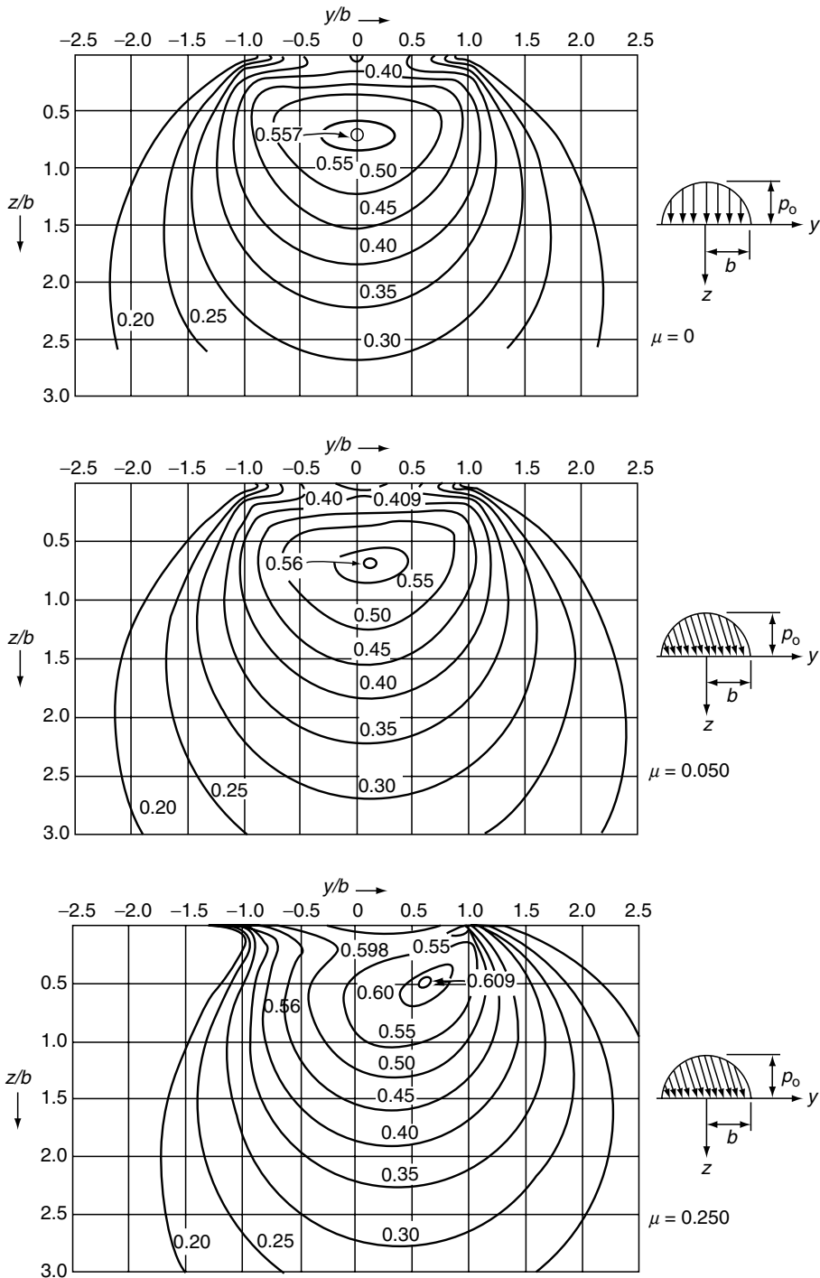
FIGURE 6.18 Lines of equal von Mises stress/normal applied stress for various surface shear stresses \tau /normal applied stress \sigma . (From Zwirlein, O. and Schlicht, H., Werkstoffanstrengung bei Wälzbeanspruchung-Einfluss von Reibung und Eigenspannungen , Z. Werkstofftech. , 11, 1–14, 1980.)
