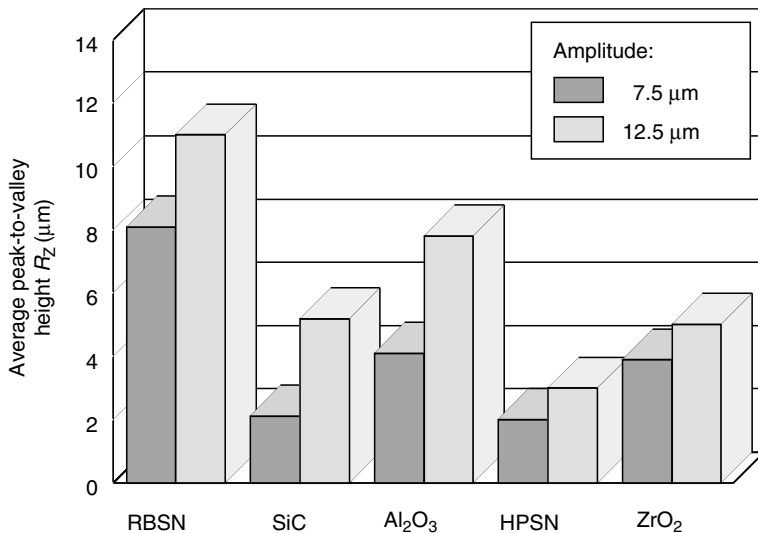
FIGURE 17.7 Relation of surface quality and amplitude of shape-generating counterpart (abrasive: \text{B}_4\text{C} F320, 50 Vol.%). (From Haas, R., Verfahren zur dreidimensionalen Bearbeitung keramischer Werkstoffe. Werkstoffe und Konstruktion 2, 2, Germany, S127–133, 1988.)
