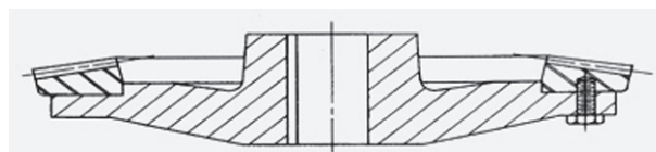
a) Webless-type wheel
