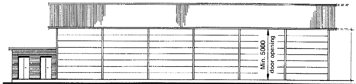
ELEVATION
