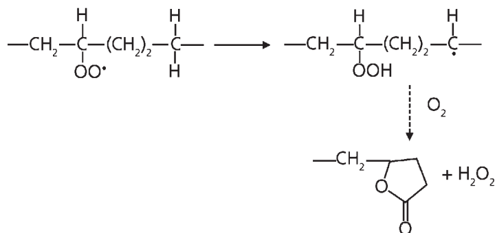
Scheme 10.14
