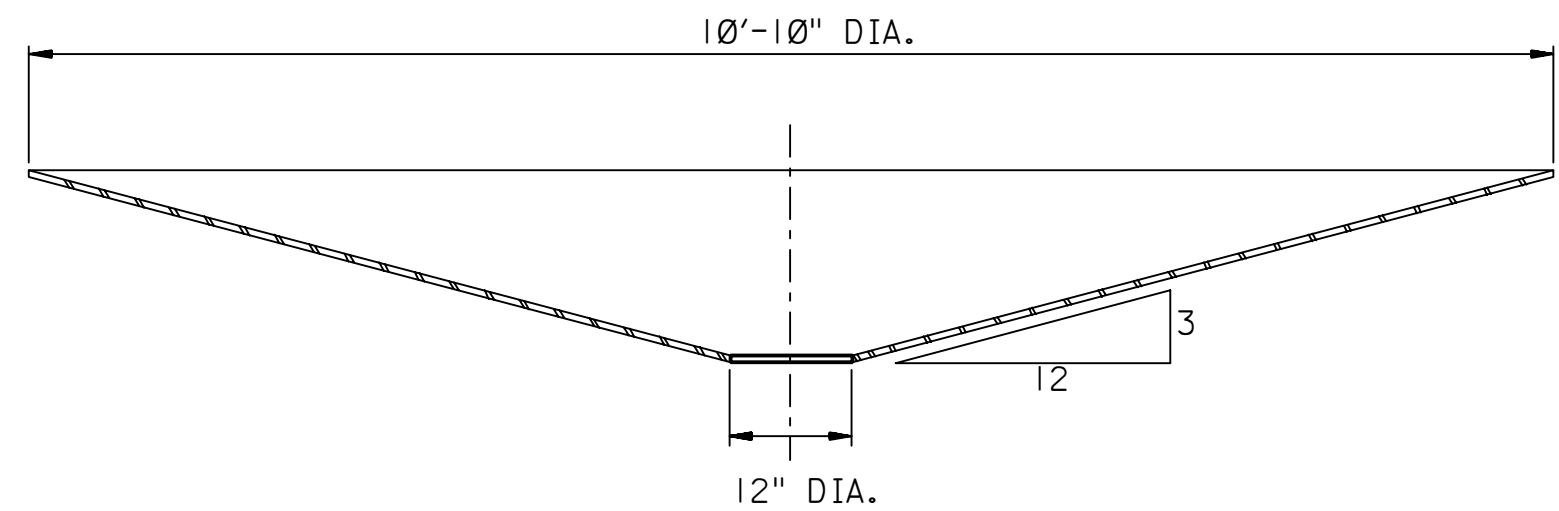
SECTION A-A
