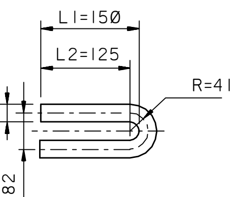
DETAIL 6 (TYP.)
