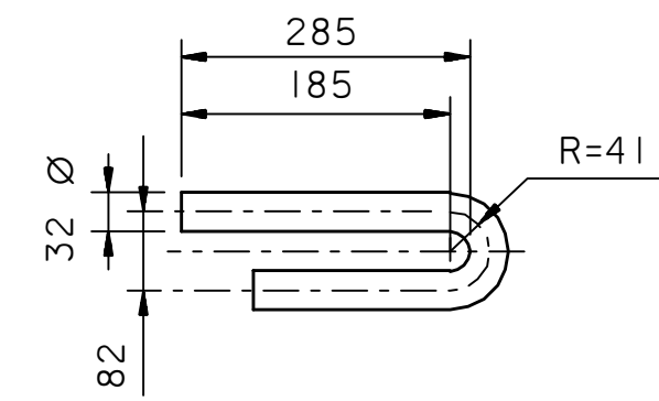
DETAIL 7 (TYP.)
