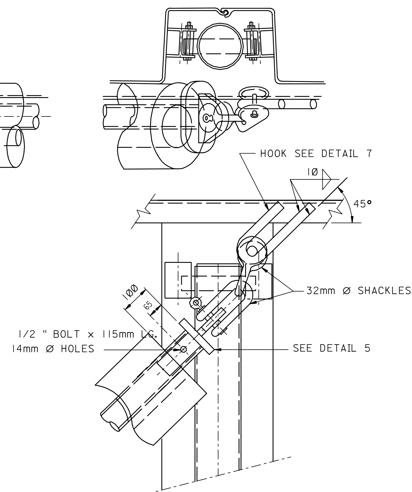
DETAIL 4 (TYP.)
