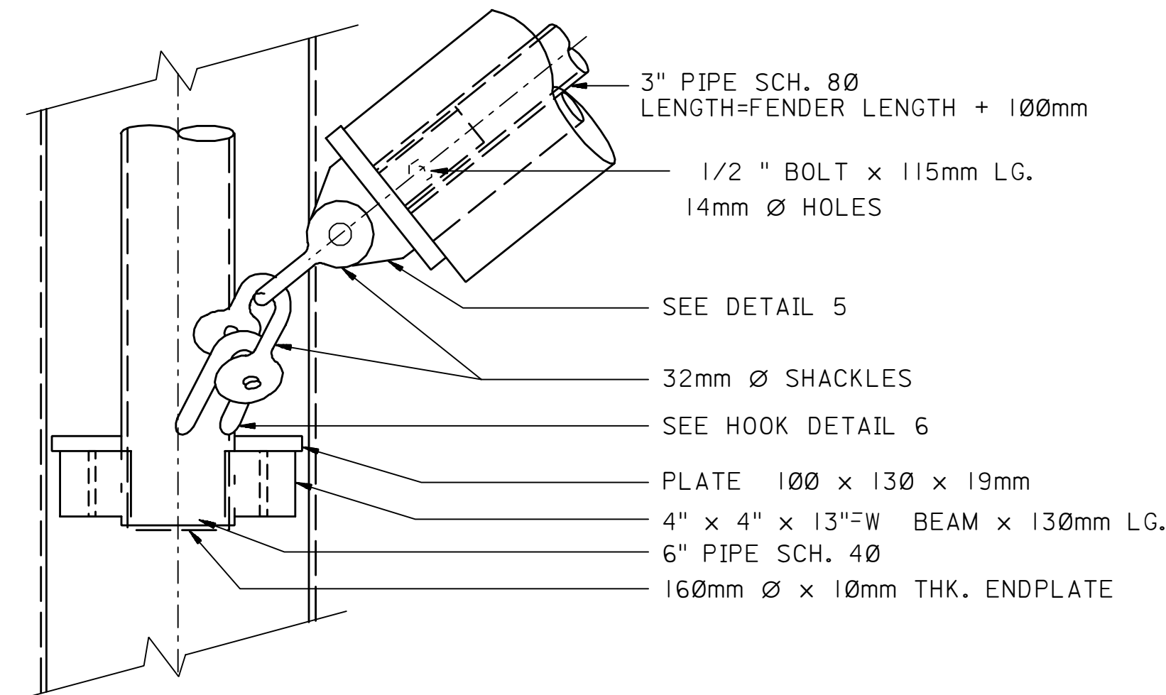
DETAIL-2 (TYP.)
