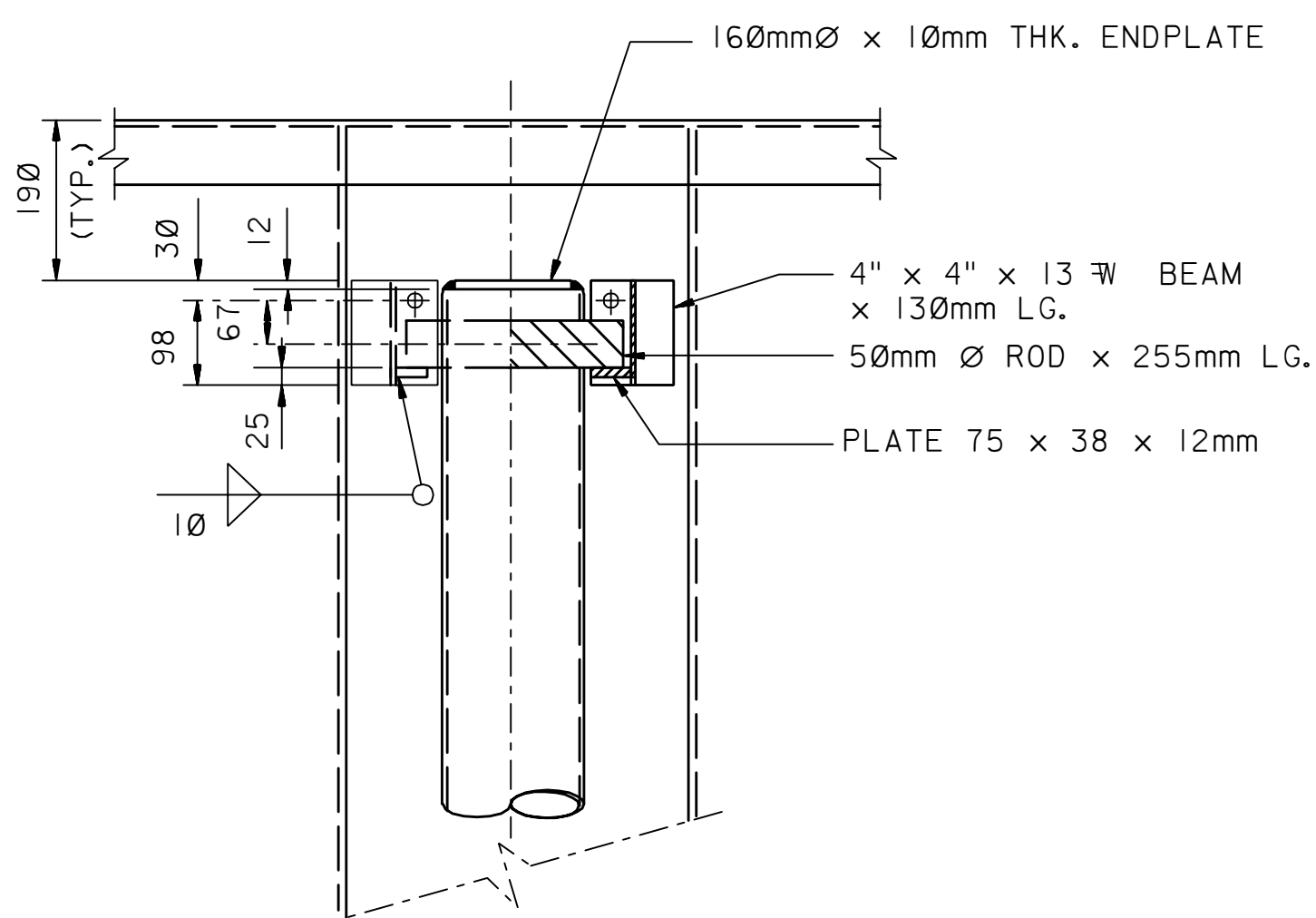
DETAIL-1 (TYP.)
